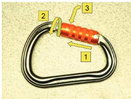
Bild 12: HMS-Karabinerhaken mit drei voneinander unabhängigen Bewegungen zum Öffnen des Schnappers (sog. „Redundanzkarabiner“). (Quelle: Werft)
