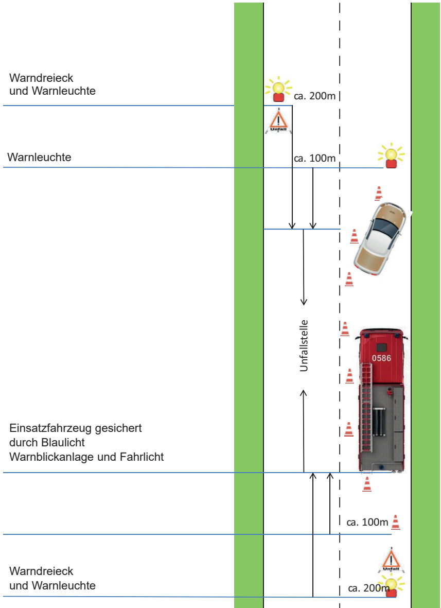
Bild 4: Absichern von Einsatzstellen auf Straßen außerhalb geschlossener Ortschaften nach (GUV-I 8651)
