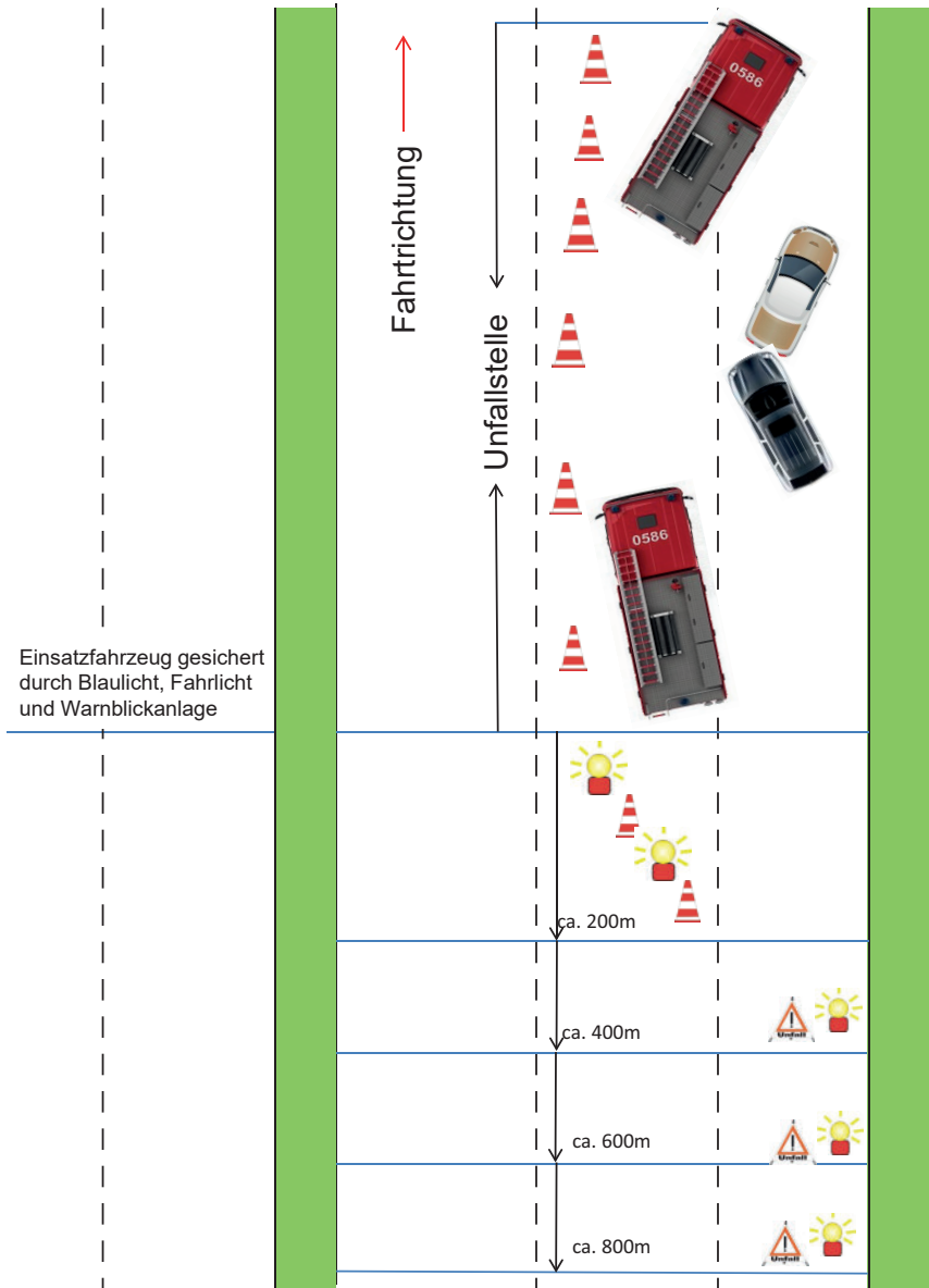
Bild 5: Absichern von Einsatzstelle auf Autobahnen nach (GUV-I 8651)
